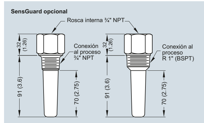
SensGuard opcional, dimensiones en mm (inch)
