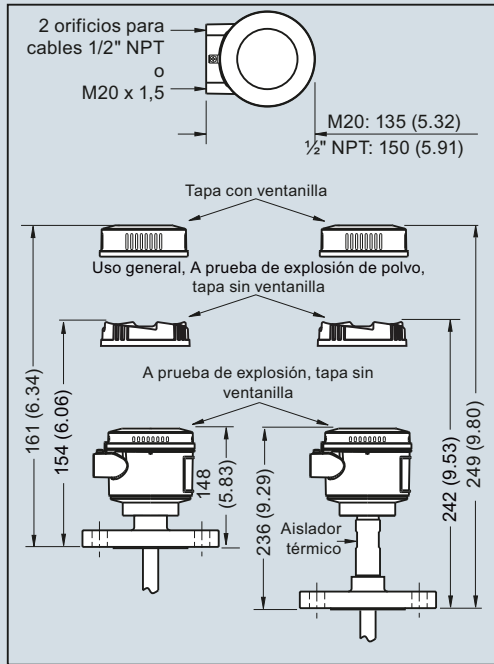
Pointek CLS200 conexiones de proceso bridadas, dimensiones en mm (inch)
